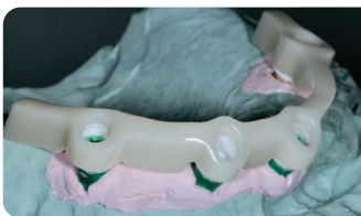
Reduzierter Steg aus Vollzirkon verklebt mit den Abutments auf dem Modell in situ
